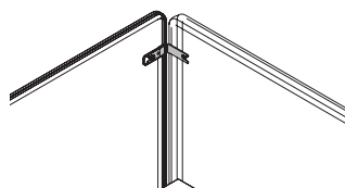
T-Panel Curve monté dans la découpe du plateau (un cache en matière plastique pour la découpe du plateau n'est pas disponible)
