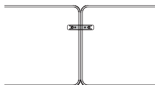
T-Panel Curve assemblage en ligne éléments de liaison : SZ noir
