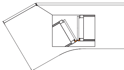
vue détaillée du joint de finition souple lors d'une disposition en rang
