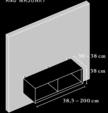
KB BOX AN WAND UND MAUERWERK KB BOX ON THE WALL AND MASONRY
