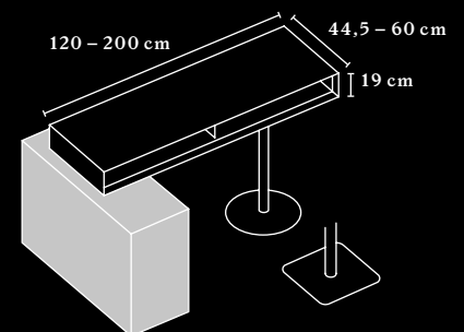
KB BOX STEHTISCH AUFGESETZT AUF SCHRANK KB BOX, HIGH TABLE MOUNTED ON THE CABINET
