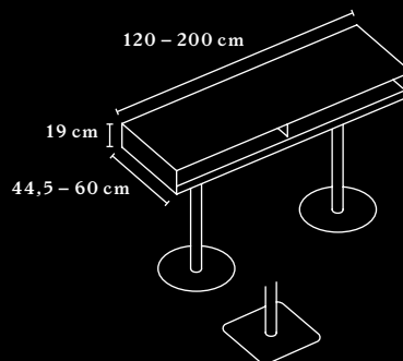
KB BOX STEHTISCH KB BOX HIGH TABLE
