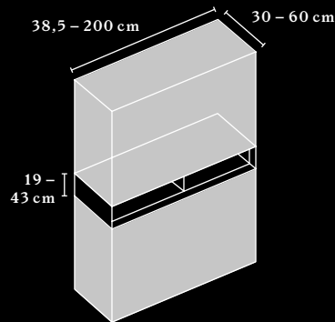
KB BOX ZWISCHEN 2 SCHRÄNKEN INTEGRIERT KB BOX INTEGRATED BETWEEN TWO CABINETS
