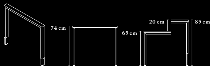
RECHTECKROHR 1 RECTANGULAR PIPE 1
