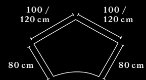
WINKELTISCH GLEICHSEITIG 120° EQUAL-SIDED 120° ANGLE DESK
