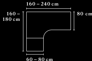
KOMBITISCH K3 COMBINATION DESK K3
