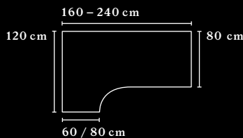
KOMBITISCH K1 COMBINATION DESK K1
